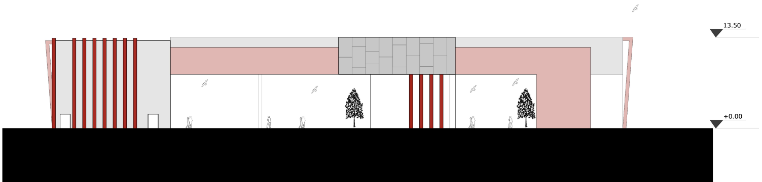
GÜNEY CEPHESİ Ö:1/200
