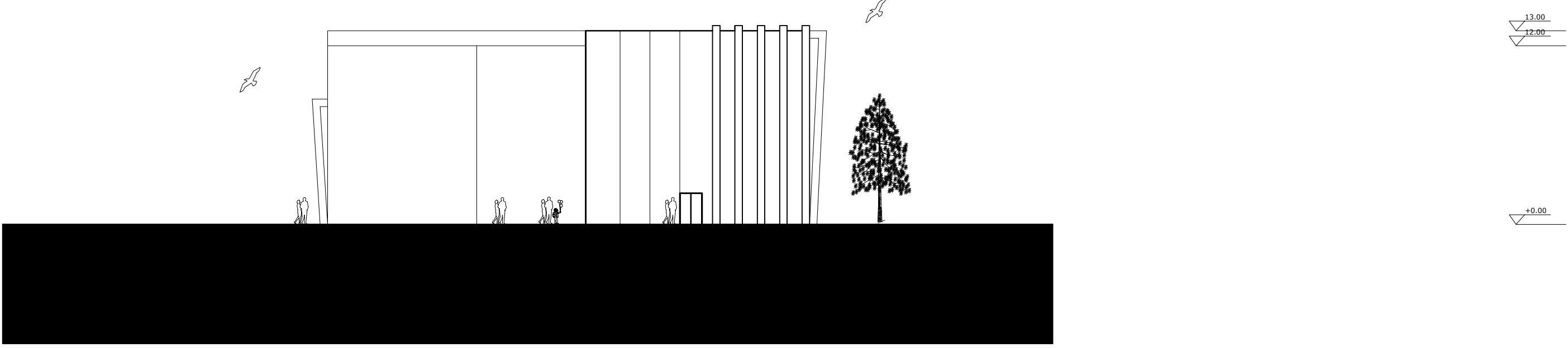
DOĞU CEPHESİ Ö:1/200
